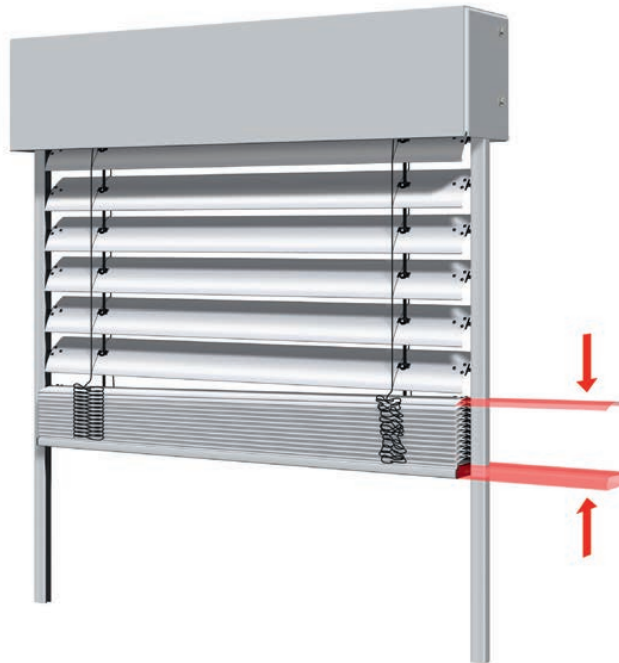
Bild 11: Paketparallelität (Lamellenpaket schief, Unterschiene gerade)
