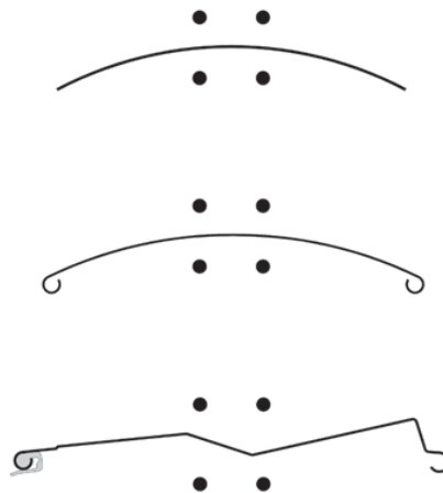
Bild 3: Sichtflächendefinition gängiger Raffstorelamellen
