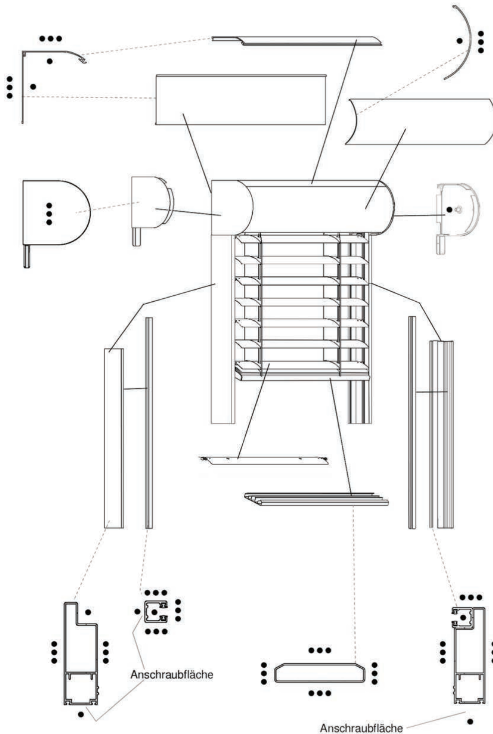
Bild 2: Sichtflächendefinition – Vorbauraffstore
