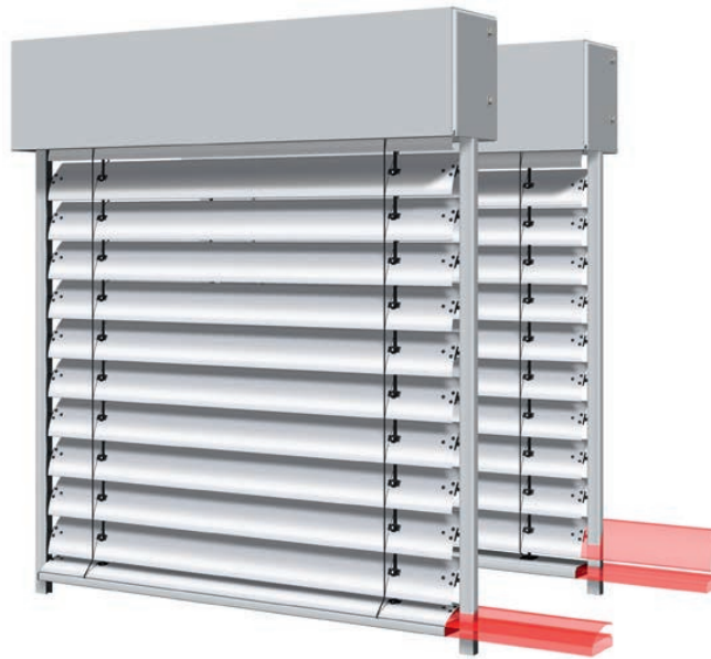
Bild 12: Teilungsausgleich
