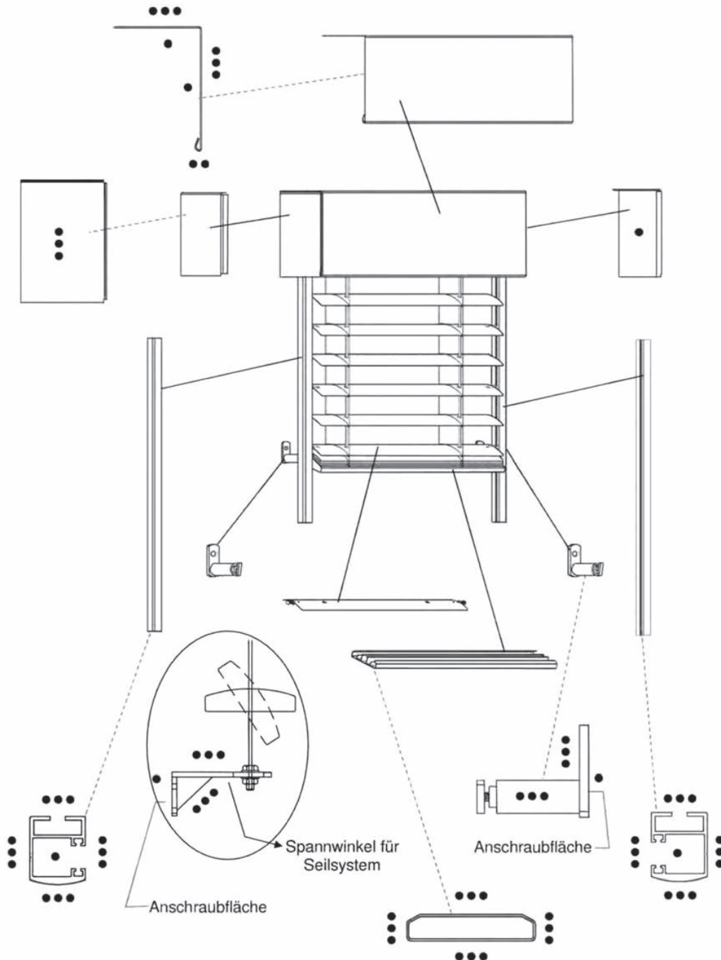
Bild 1: Sichtflächendefinition – Raffstore mit Blende
